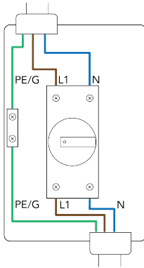
Ligação monofásica
